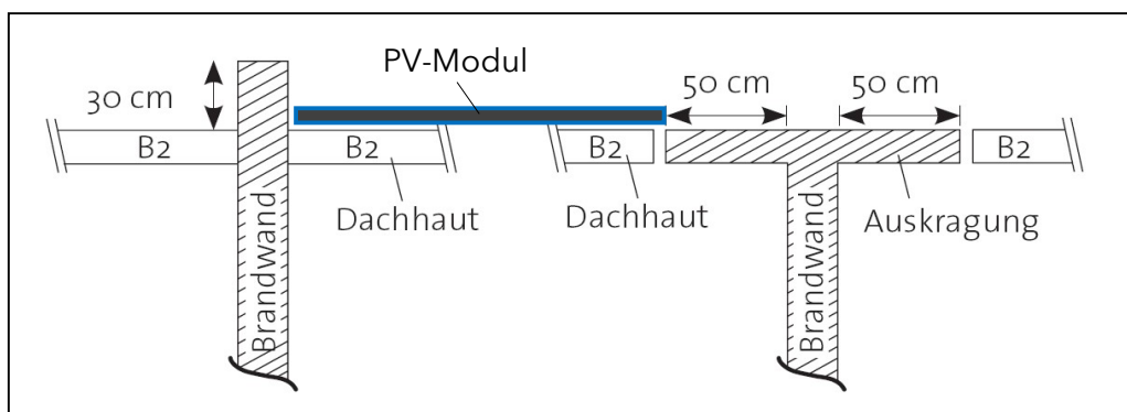
Abbildung 5: Mögliche Ausführungen einer Brandwand; Anordnung von dachparallelen PV-Modulen direkt an der über das Dach geführten Brandwand oder mit Abstand bei der Brandwand mit Auskragung
